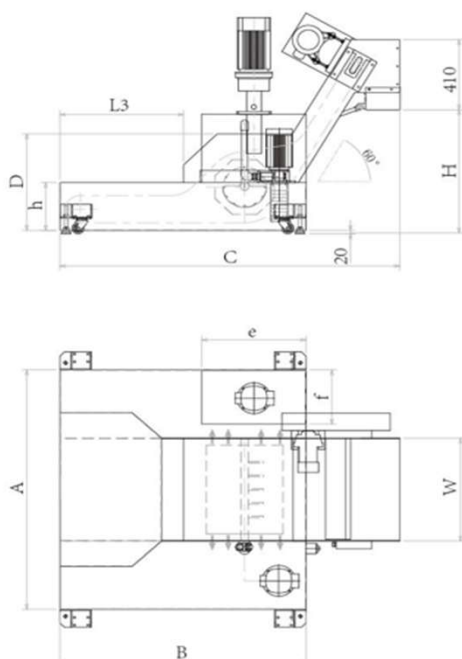
外形図 Outline Drawing
